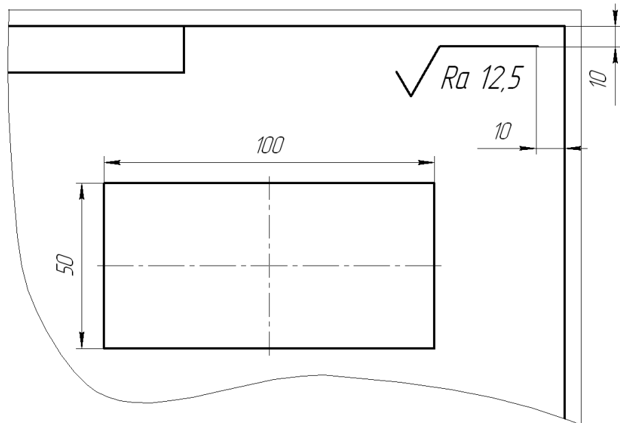
Рисунок 5.4 – Всі поверхні деталі мають однакову шорсткість
