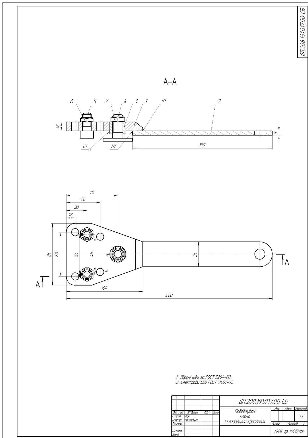
Рисунок 5.20 – Приклад складального креслення
