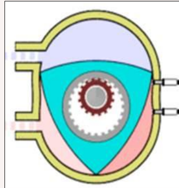
Двигун Ванкеля
