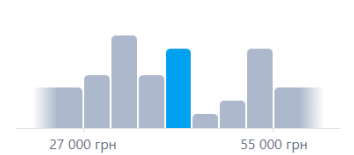
Розподіл зарплат
