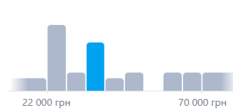
Розподіл зарплат
