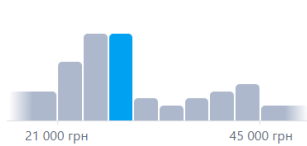
Розподіл зарплат
